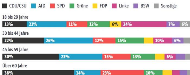
Рисунок 3: Решение о голосовании в зависимости от возраста
